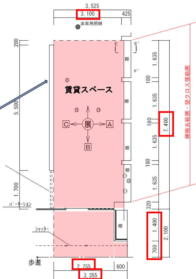
平面图 S=1 : 100
