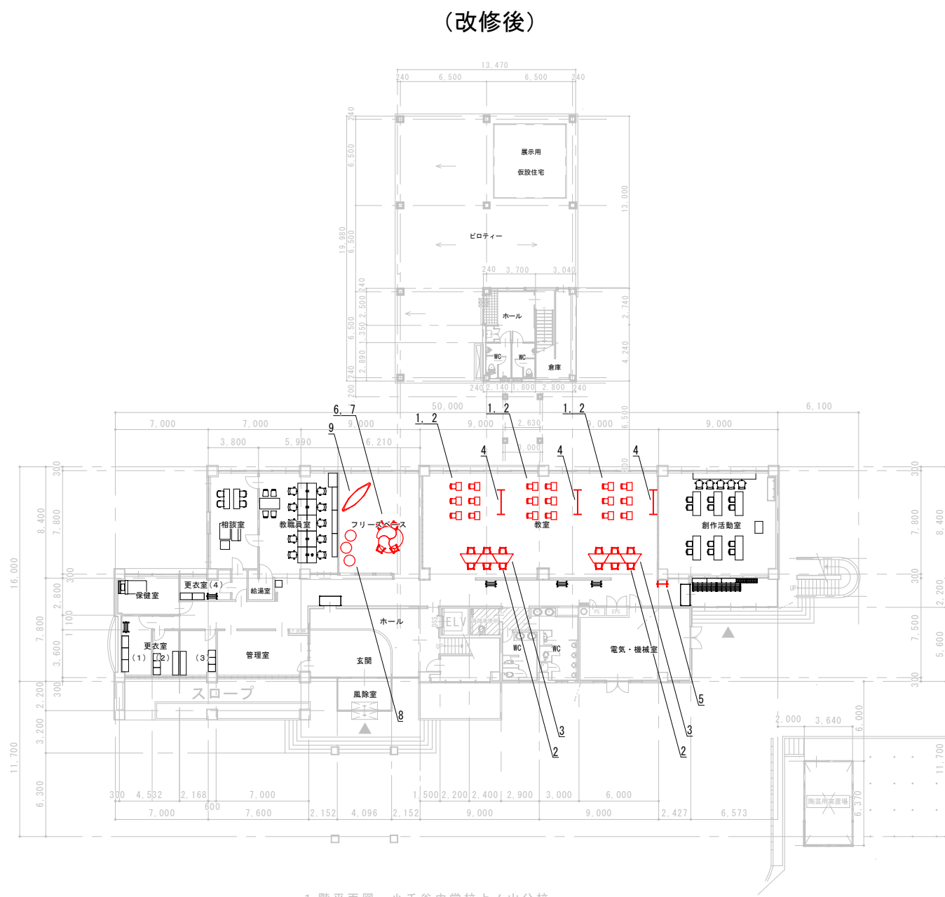
1 階平面図 小千谷中学校上ノ山分校
