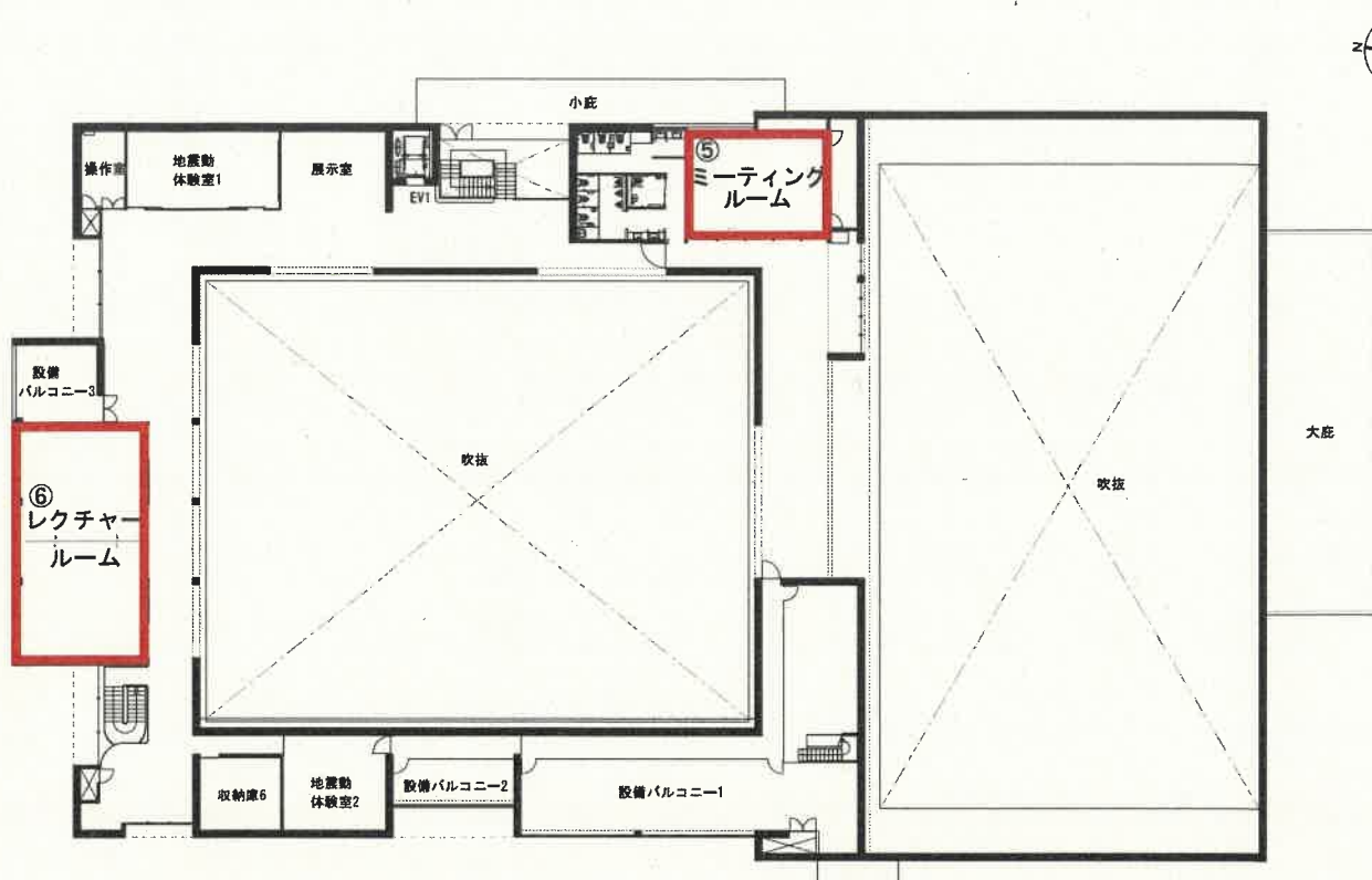
2階平面図 S=1/600
