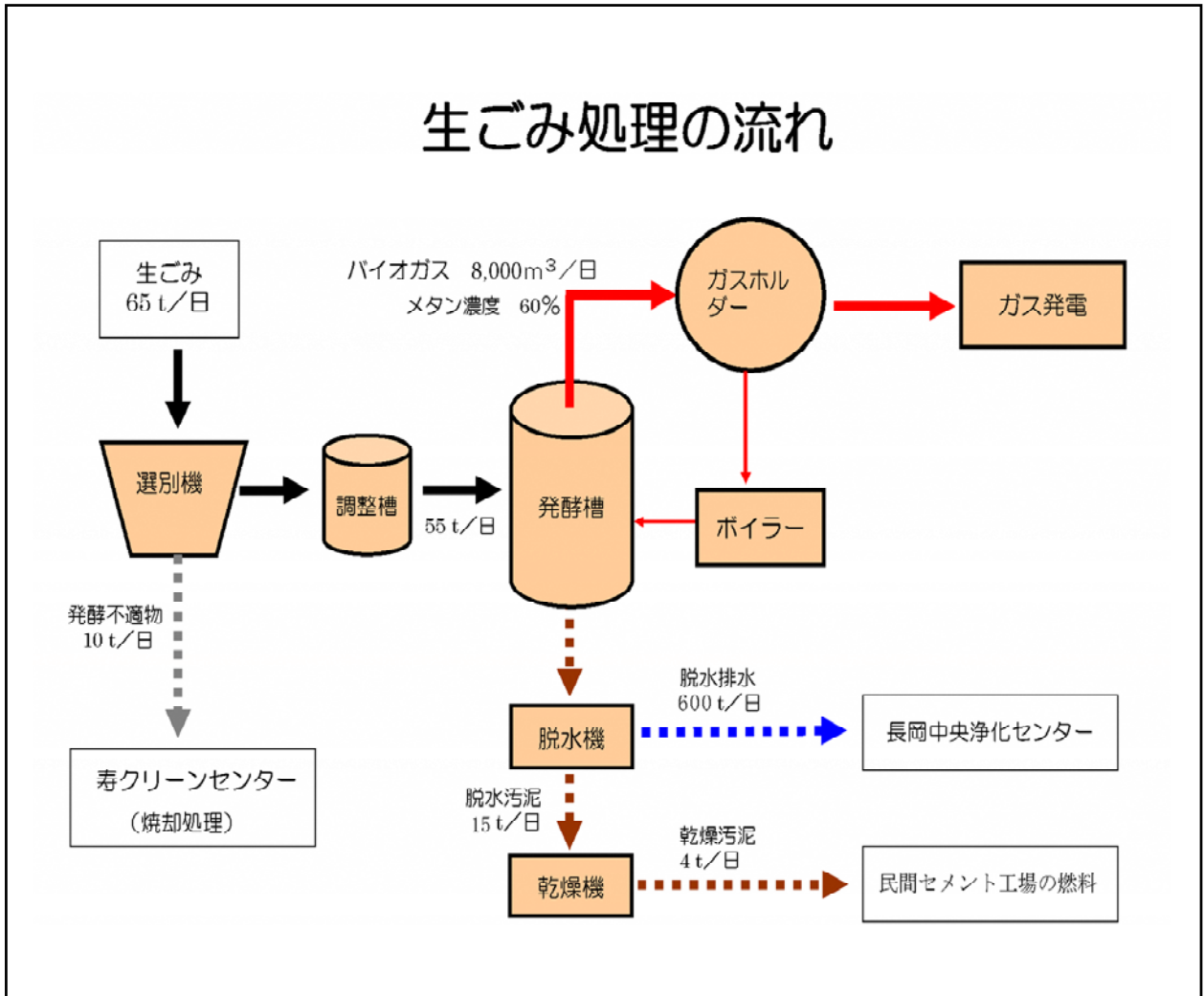
図 生ごみバイオガス化施設による生ごみ処理のイメージ 出典：長岡市環境施設課
